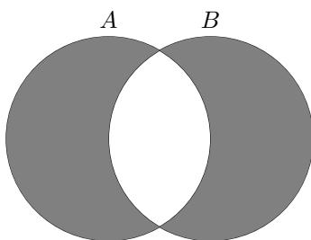
FIGURA 3.24 Differenza simmetrica tra insiemi (ombreggiata).
