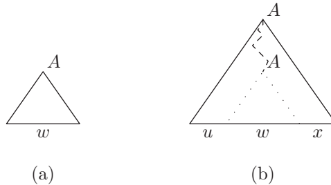
FIGURA 4.3 (a) sottoalbero che genera w . (b) sottoalbero che genera vw .
