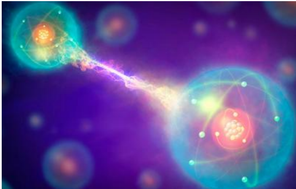
Entanglement quantistico
